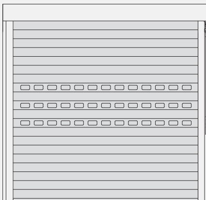
Vrata z profilů AW 100 (příklad prosklení - pohled zevnitř)
